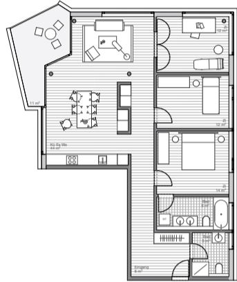
4 1/2 Zimmerwohnung (107 m²) Haus A 1:100
