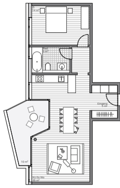
2 1/2 Zimmerwohnung (82 m²) Haus A 1:100
