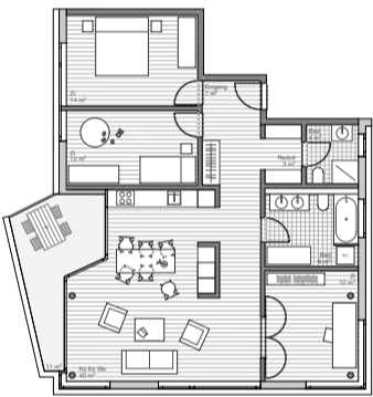
4 1/2 Zimmerwohnung (100 m²) Häuser B und C 1:100
